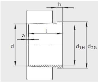
AH240、AH241 锥度为 1：30
